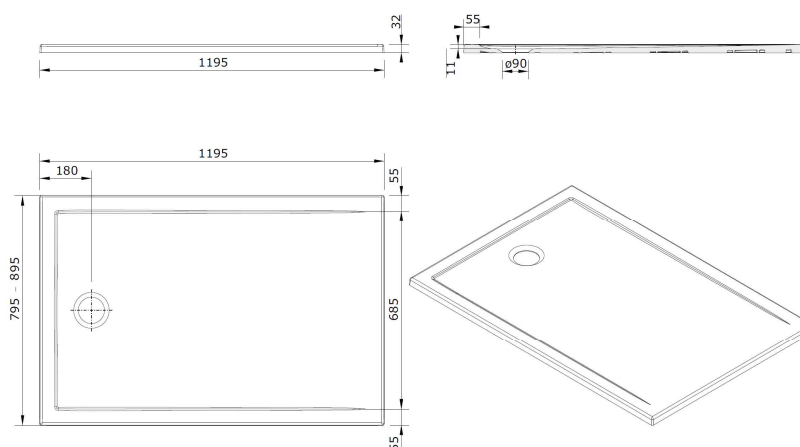
Receveur de douche Step-In en 120 x 90 cm
